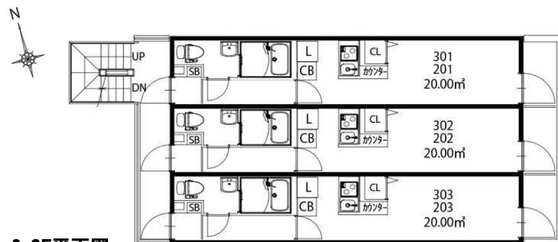
2・3F平面図
